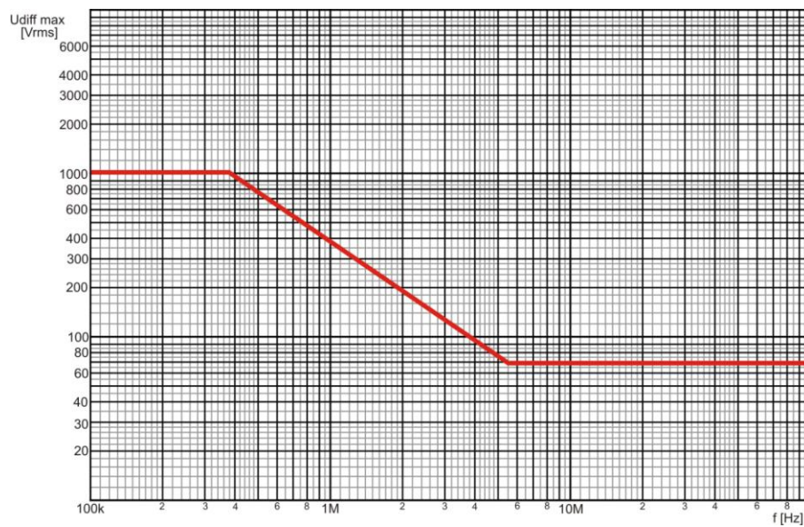
Obr. 3.2. Závislosť maximálnej hodnoty diferenciálneho vstupného napätia od frekvencie.
