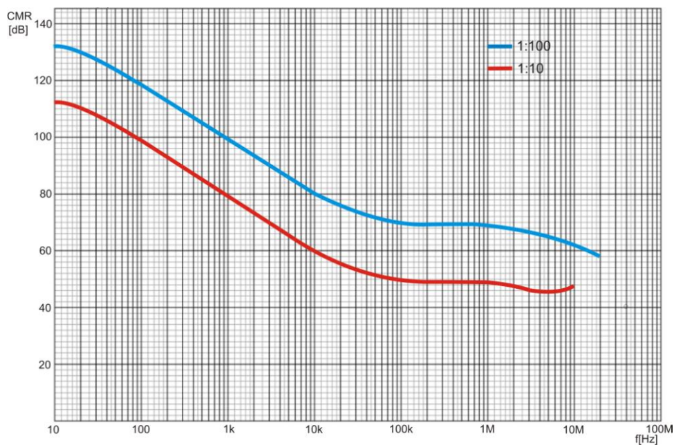
Obr. 3.1. Typická závislosť CMR na frekvencii
